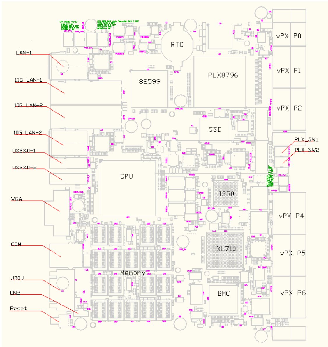
图 3-1 VPX-S6B02 TOP 面接口图
